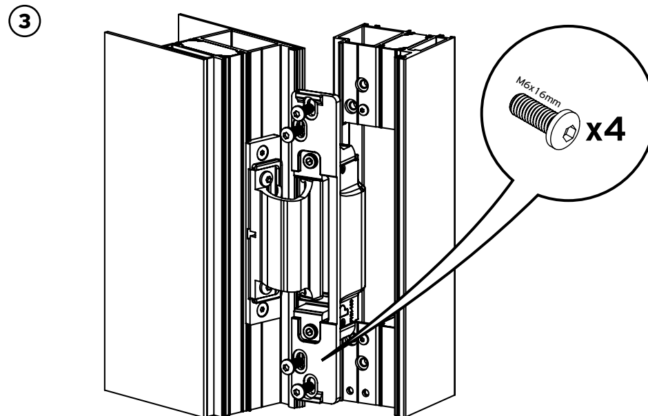
Τοποθέτηση του μεντεσέ στην κάσσα.
