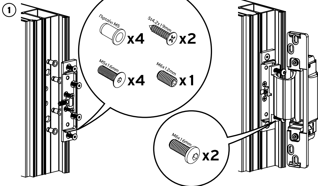
Τοποθέτηση του μεντεσέ στο φύλλο.
