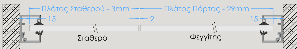
ΤΟΜΗ Κ-Κ
