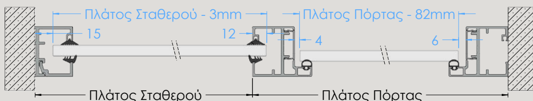
ΤΟΜΗ Η-Η
