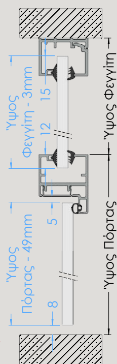
ΤΟΜΗ Β-Β
