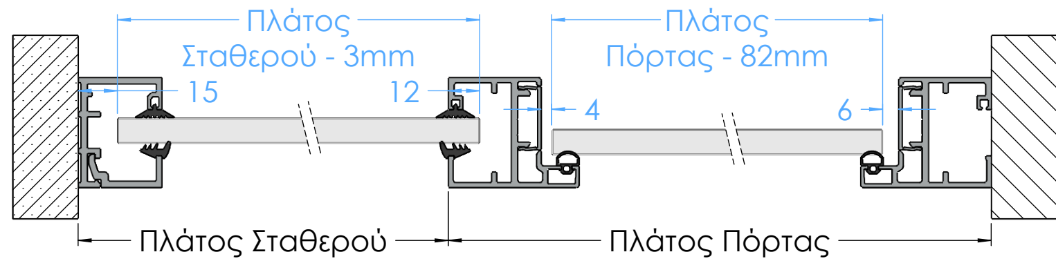
ΤΟΜΗ K-K
