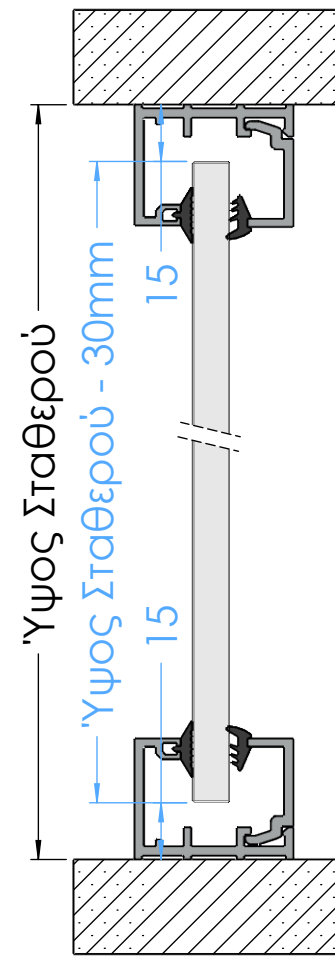
ΤΟΜΗ Α-Α
